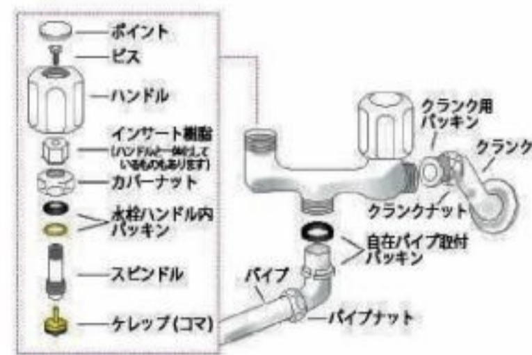
雙付き2ハンドル混合栓の構造
